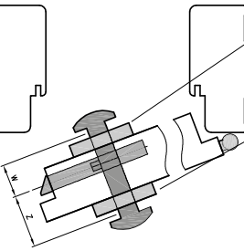
Pav. Cilindro su rankena dydžio pasirinkimas
