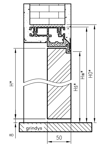
50 mm durų su apversta užlaida – atsidarančių į vidų, vertikalus pjūvis
