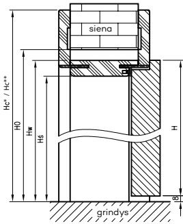
Vertikalūs pjūvis OR
