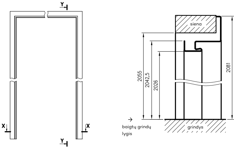
matmenys vienvėrems durims
