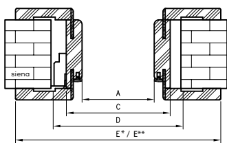
Horizontalus pjūvis OR
