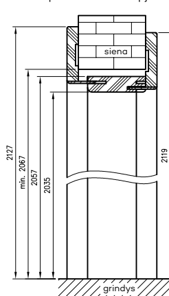
Reguliuojamo tunelio su kamp. T80 vertikalus pjūvis
