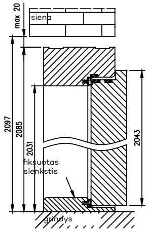
Medinė stakta „Athos“ durims su fiksuotu slenksčiu
