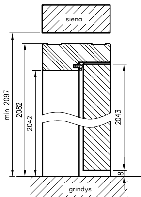
Vertikalus pjūvis OPB
