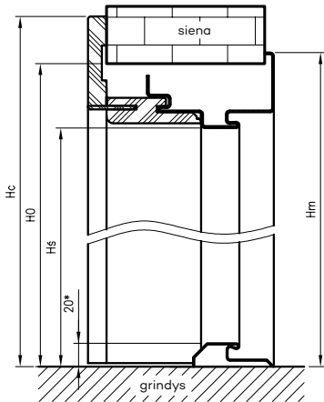
OSH STAND matmenys dvivėrėms durims
