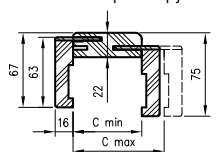
TUN su kamp. T63 pjūvis
