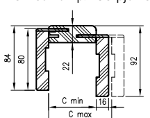
TUN su kamp. T63 pjūvis
