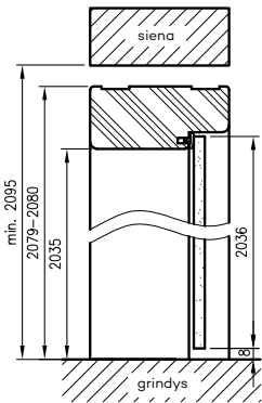
Vertikalus pjūvis OP stiklinėms durims
