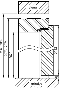
Vertikalus pjūvis OP užlaidinėms durims
