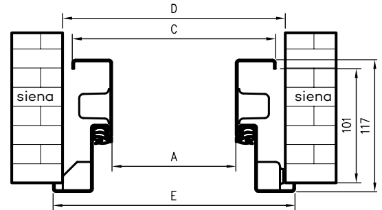
Durų staktos sienoje skerspjūvis
