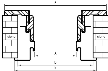
Staktos profilis
