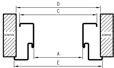
D - montavimo angos plotis
