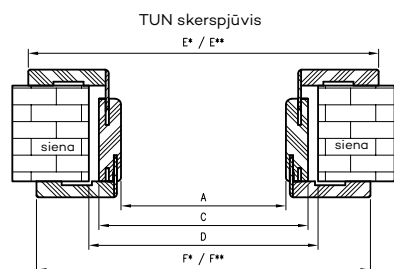
TUN su kamp. T80 pjūvis
