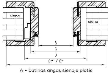
Horizontalus pjūvis OR/ORC
