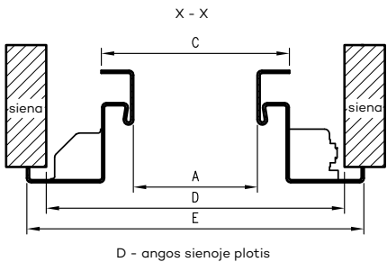
matmenys vienvėrems durims
