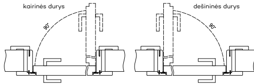
Staktos profilis
