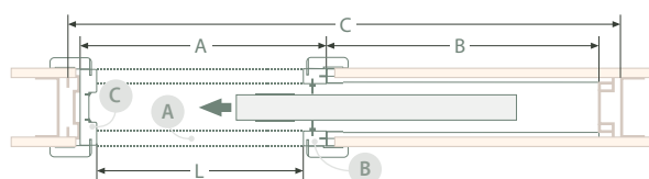
VIENVĖRĖS KASETĖS MATMENYS (mm)
