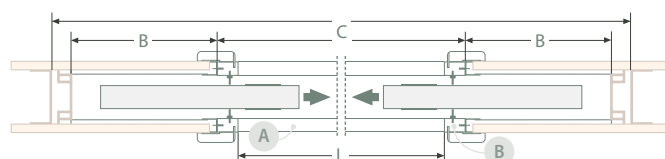
DVIGUBOS KASETĖS MATMENYS (mm)
