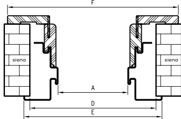
Staktos profilis
