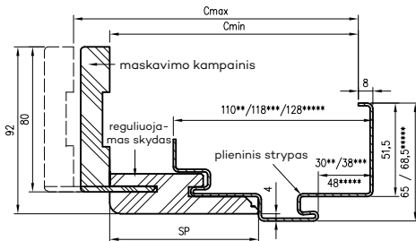
Staktos profilis
