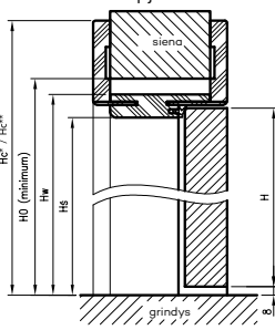
Vertikalus pjūvis ORB
