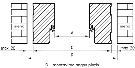
IŠ OLIMP EI30 vienvėrėms durims
