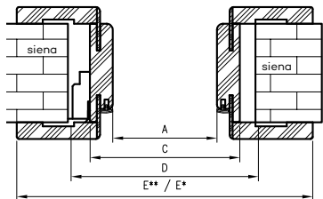
Horizontalus pjūvis OR/ORC
