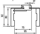
Pjūvis ORB 075
