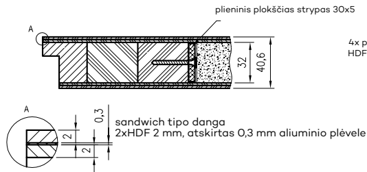
„Solid RC2“ priešįsilaužiminė durų varčia
