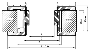
Horizontalus pjūvis ORB
