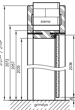
Stiklinių durų su ORC vertikalus pjūvis stiklinės durys iš ORC
