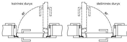
Staktos profilis
