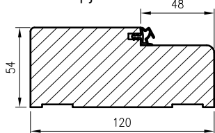
OLIMP EI60 durų medinio staktos pjūvis
