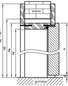
Vertikalus pjūvis OR
